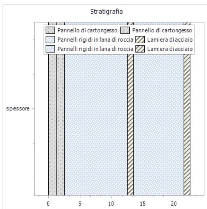
Rappresentazione stratigrafia
